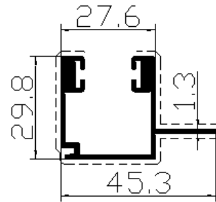
Profil No: 4934 Gramaj : 0,599 kg/mt
