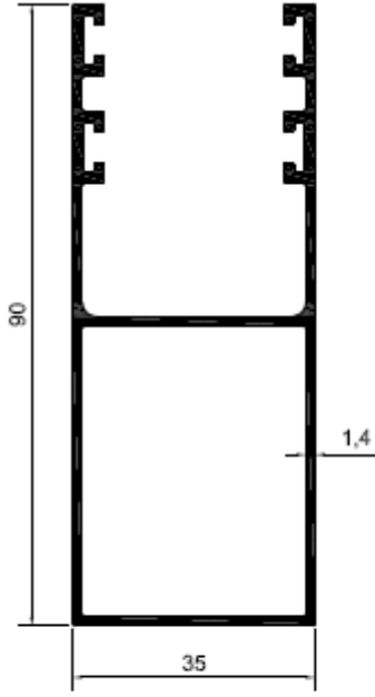
KOD-2200 TEORİK AĞIRLIK-1,109 KG/M
