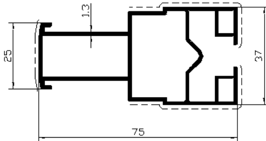
Profil No: 6050 Gramaj : 1,065 kg/mt
