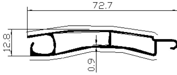
Profil No: 7123 Gramaj : 0,436 kg/mt
