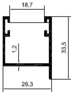
KOD-2203 TEORİK AĞIRLIK-0,331 KG/M
