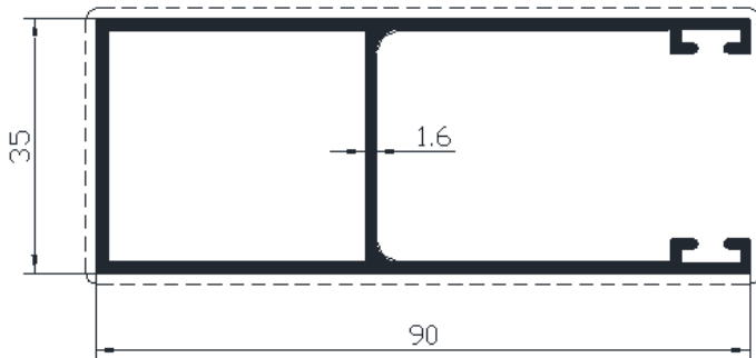
Profil No: 6953 Gramaj : 0,73 kg/mt
