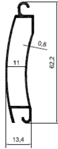
KOD-2803 TEORİK AĞIRLIK-0,358 KG/M
