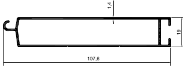
KOD-2103 TEORİK AĞIRLIK-0,949 KG/M
