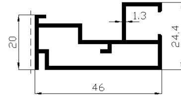
Profil No: 6079 Gramaj : 0,596 kg/mt
