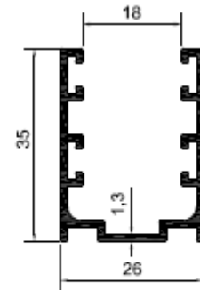
KOD-2105 TEORİK AĞIRLIK-0,466 KG/M
