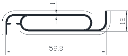
Profil No: 6980 Gramaj : 0,355 kg/mt
