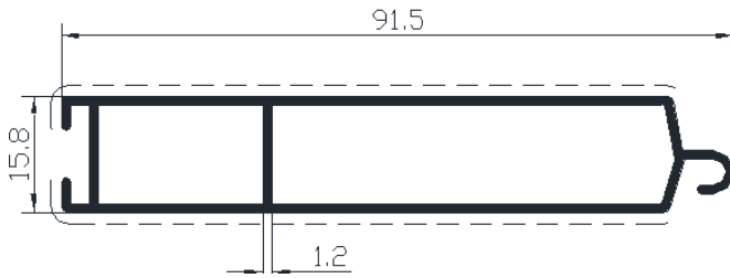
Profil No: 6953 Gramaj : 0,73 kg/mt
