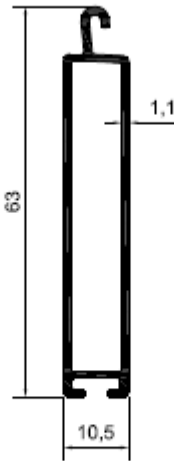
KOD-2101 TEORİK AĞIRLIK-0,434 KG/M
