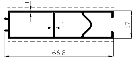
Profil No: 6991 Gramaj : 0,518 kg/mt
