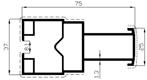
Profil No: 6133 Gramaj : 1,014 kg/mt
