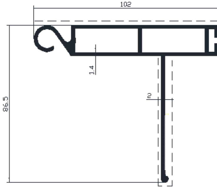
Profil No: 6345 Gramaj : 0,910 kg/mt
