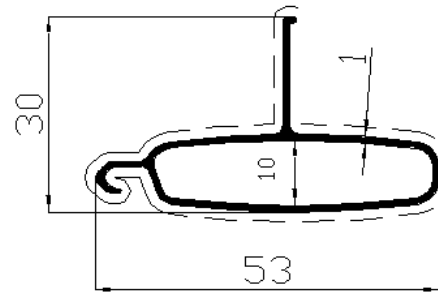
Profil No: 4435 Gramaj : 0,355 kg/mt
