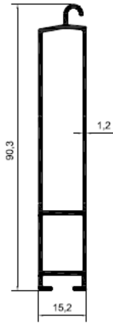
KOD-2100 TEORİK AĞIRLIK-0,724 KG/M
