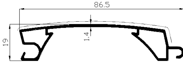
Profil No: 6345 Gramaj : 0,910 kg/mt
