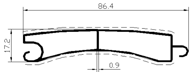
Profil No: 6952 Gramaj : 0,539 kg/mt
