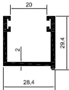
KOD-2204 TEORİK AĞIRLIK-0,480 KG/M
